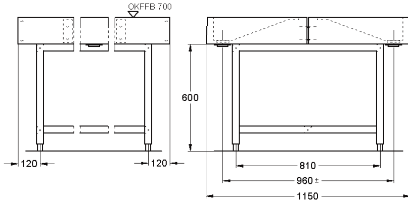
Doppelreihige Montage frei im Raum
