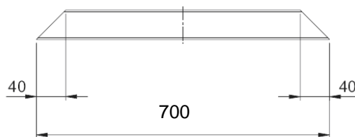
Abdeckung Trapezrinne
